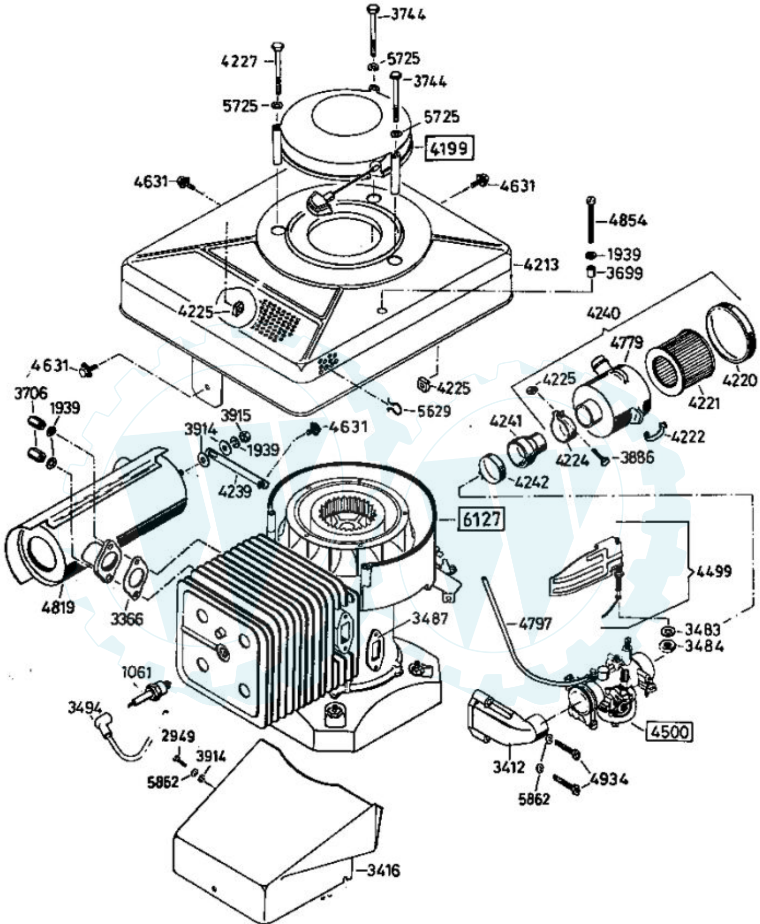
6126 Antriebsblock driving unit moteur complet
